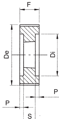
ESECUZIONE 6
