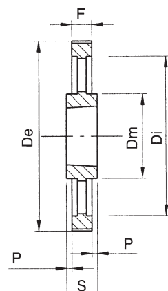
ESECUZIONE 13
