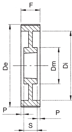
ESECUZIONE 8
