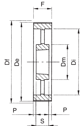
ESECUZIONE 10
