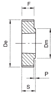
ESECUZIONE 3
