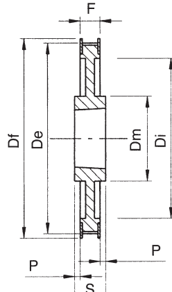
ESECUZIONE 12F
