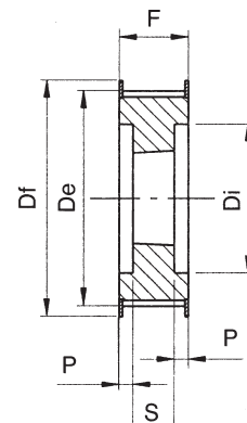
ESECUZIONE 7F
